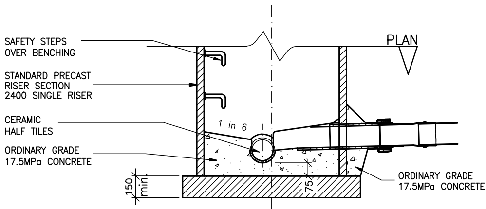
MANHOLE - PART SECTION (SD5.1) N.T.S.
