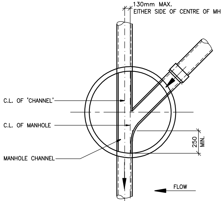
MANHOLE - PLAN VIEW N.T.S.
