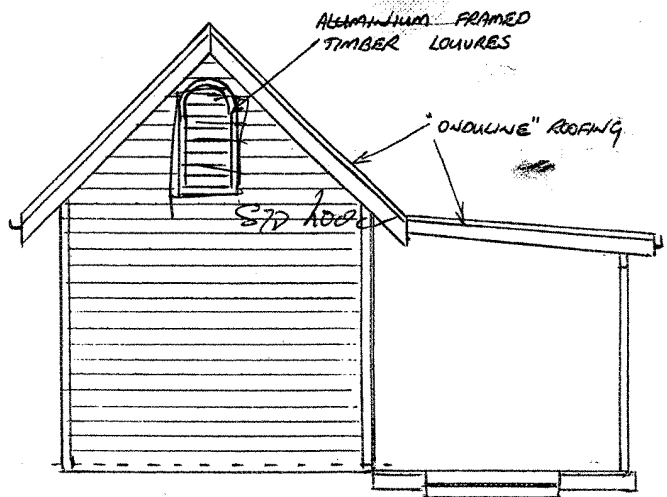
END ELEVATION
